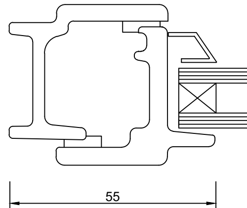
Door Section
